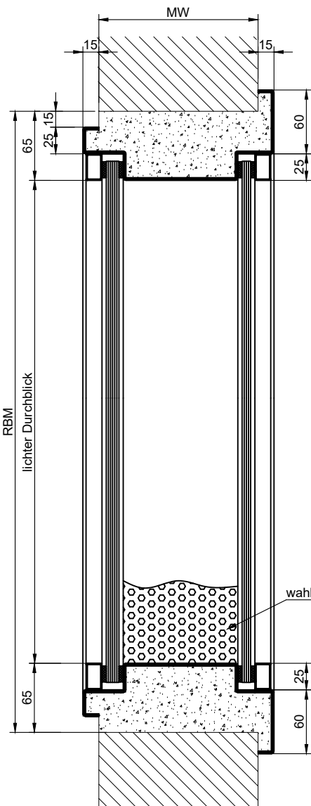
Umfassungszarge
