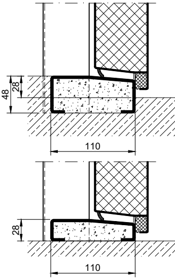
Halbschwelle
