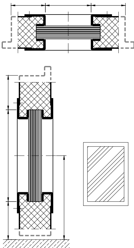
Verglasung
