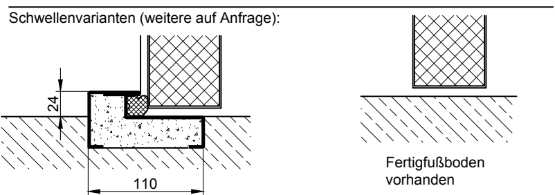
Anschlagschwelle mit Dichtungsprofil
